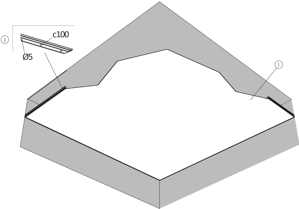
Schemat montażu (M569) dla Clipso SO Classic, montaż sufitowy z profilami PCW
