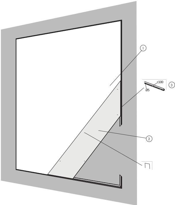
Schemat instalacji (M570) dla Clipso SO Classic, montaż ścienny
